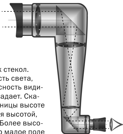
▲ Схема перископа подводной лодки
