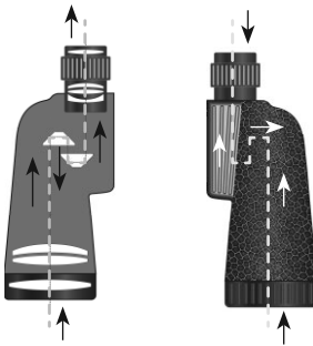
▲ Призмальный бинокль
